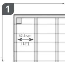
INSTALLATION BASIQUE 40,6 cm (16") DE LA SOUS-STRUCTURE
