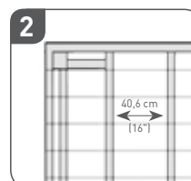
INSTALLATION AVEC ENCADREMENT DE LA SOUS-STRUCTURE
