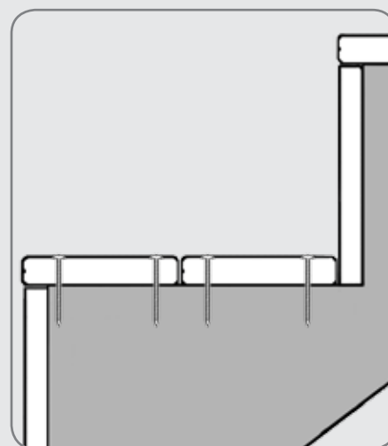
Pose basique d'un escalier
